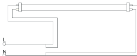
Схема підключення LB-247
