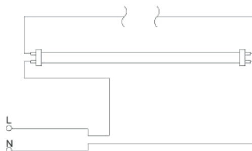
Схема підключення LB-247
