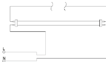
Схема підключення LB-247
