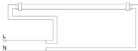
Схема підключення LB-247
