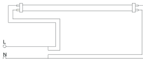
Схема підключення LB-247
